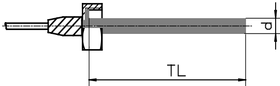
Stem type F4 union nut
