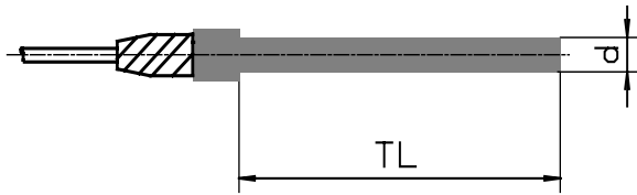
Stem type F1 plain stem without thread
